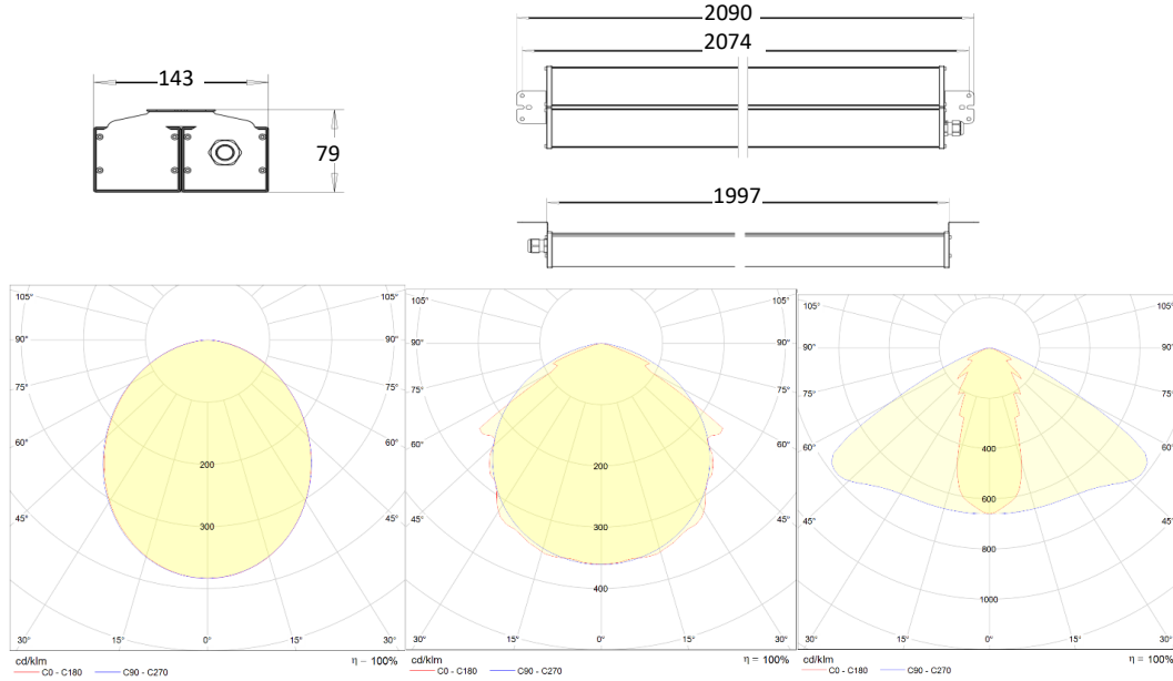
Opaalikuvun valonjako
